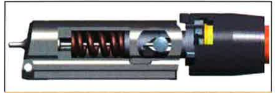
Az új konstrukciójú zártest, a Kinematic Drive szerkezete
